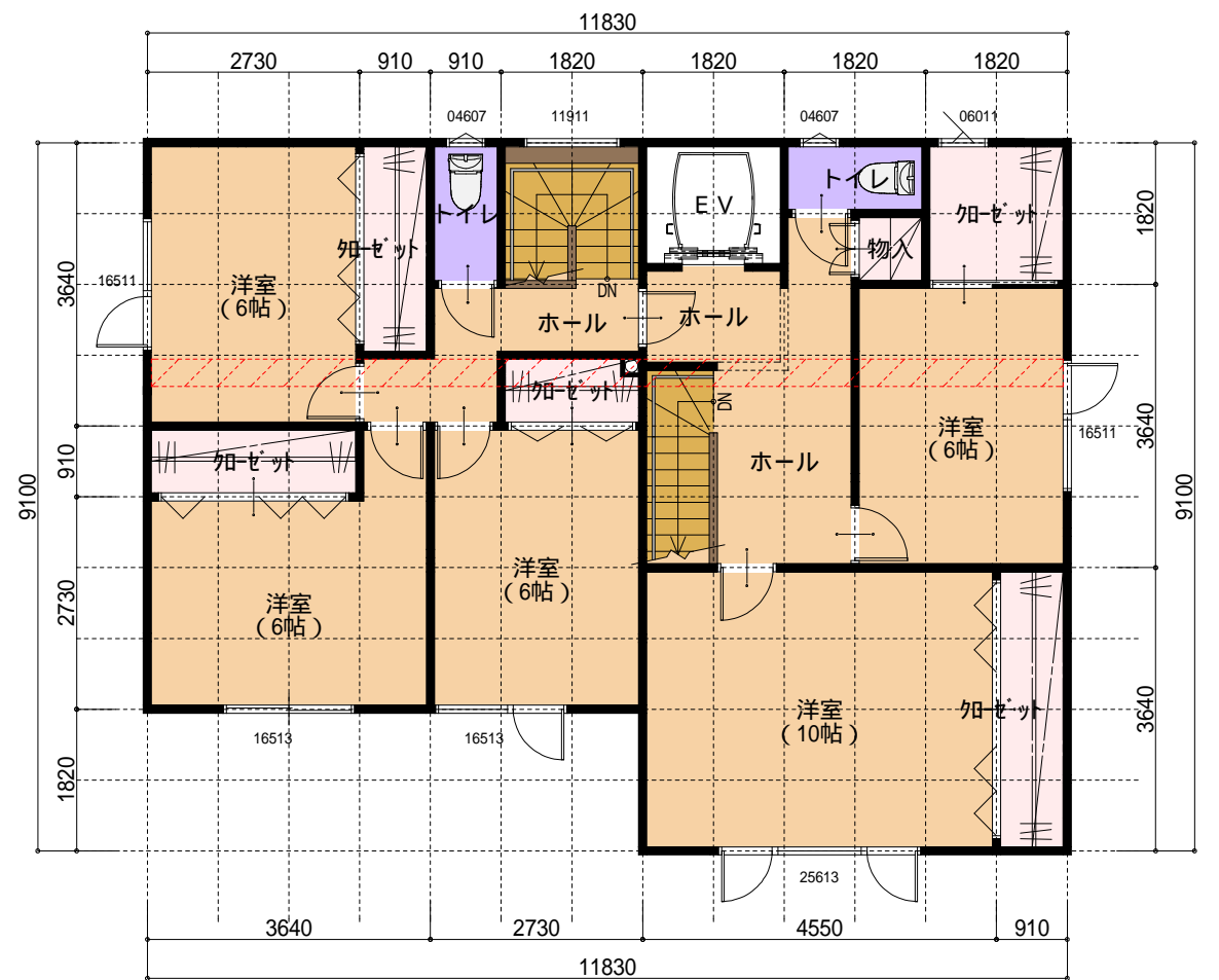
3階 平面図 S:1/100
